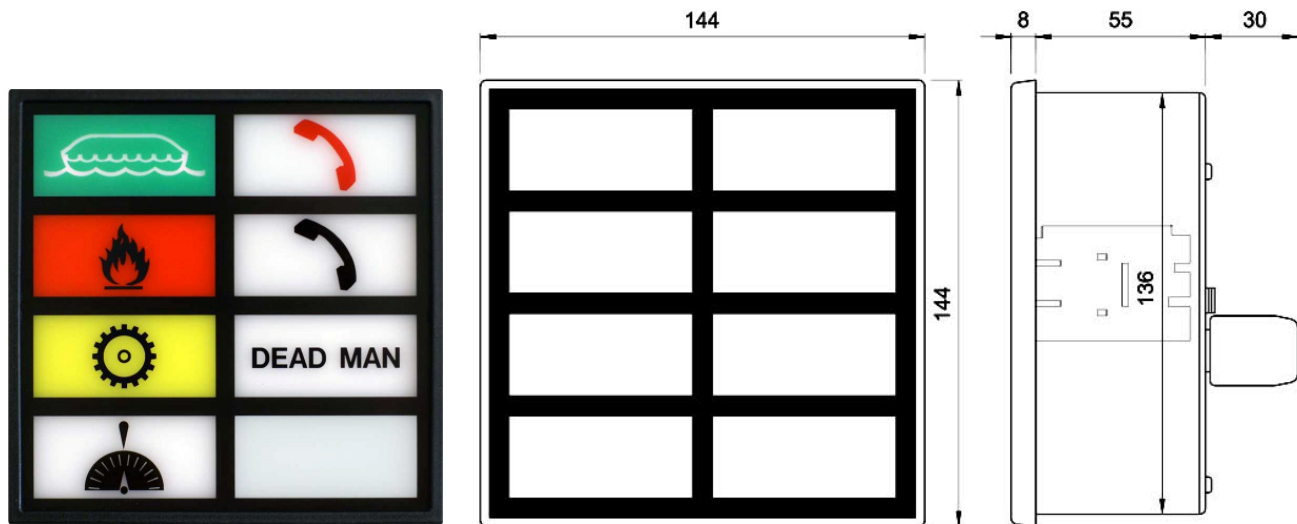
Cut-Out / Einbauausschnitt : 138 x 138 mm
